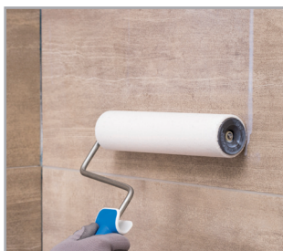
Nanošenje protukliznog zaštitnog premaza Mapecoat 4 LVT.
