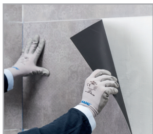
Polaganje LVT ploče na zid ljepljom Ultrabond Eco MS 4 LVT Wall.
